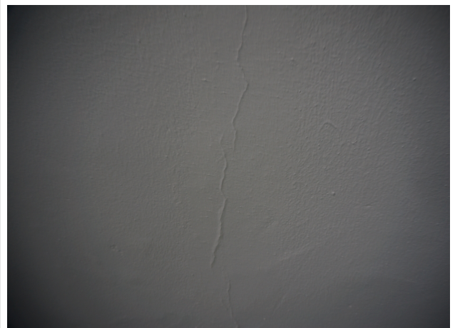
펌프실 지하1층 벽체 균열(0.3mm미만)
