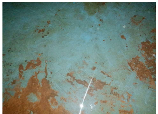
흡수정 1지 하부슬래브 도장박리
