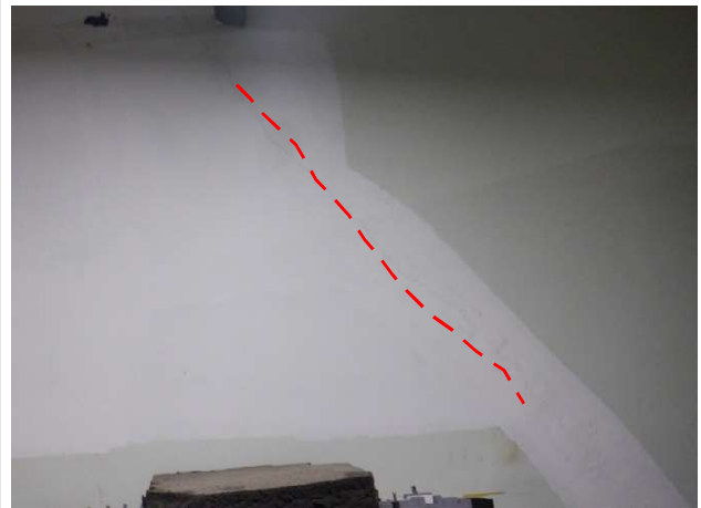
건축물 지상1층 내부 벽체(0.3mm미만)
